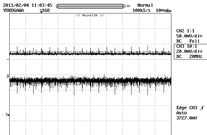
電源とLの間に抵抗(100Ω)を追加 →電圧の急激な落ち込みが無くなる
