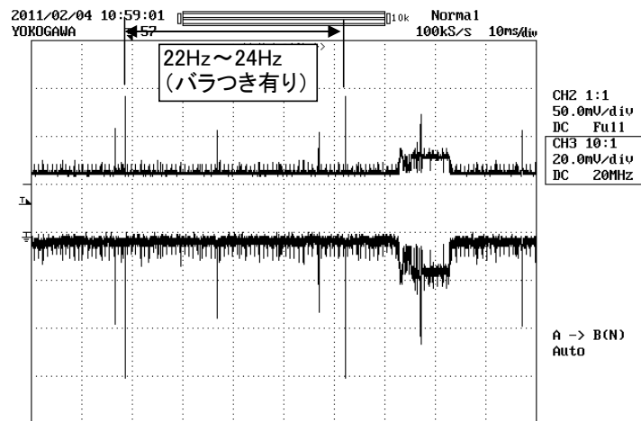
現状回路でのBattery電圧落ち込みタイミング
