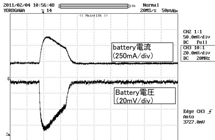
現状回路でのBattery電圧落ち込み波形
