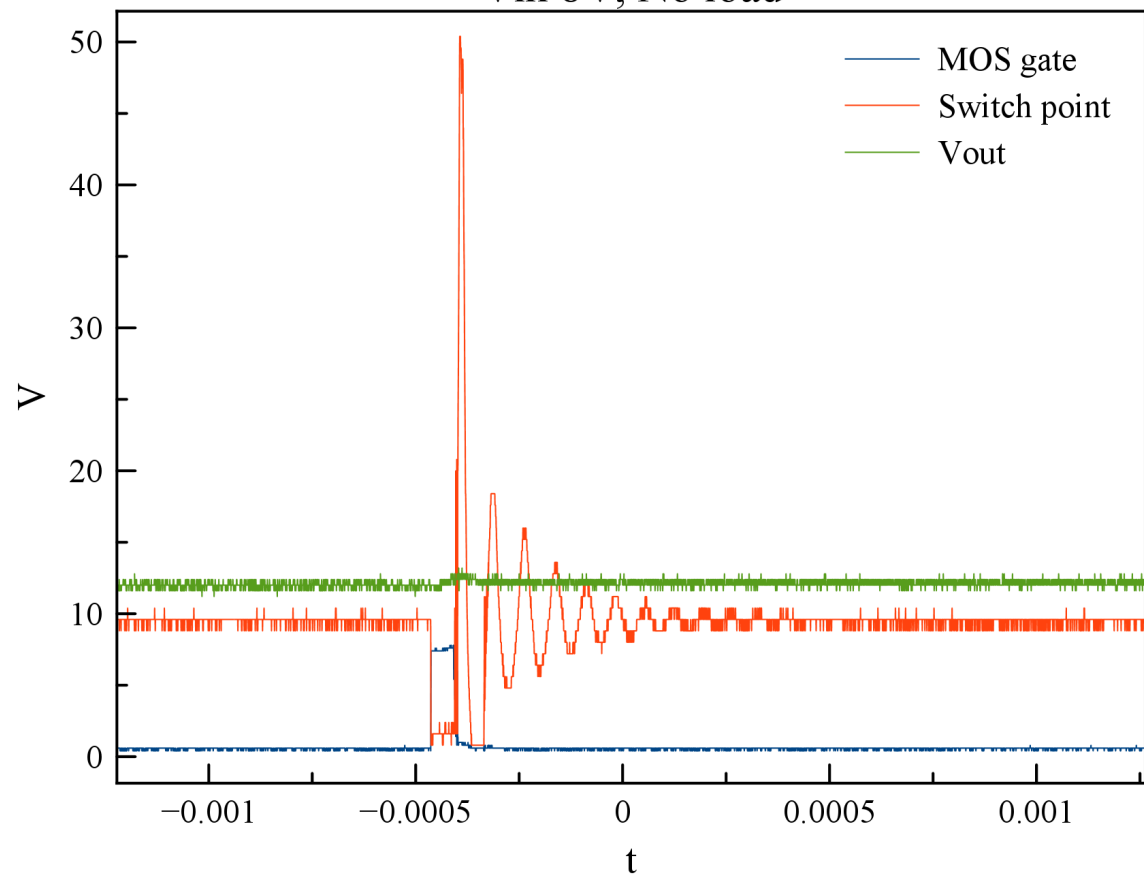
Vin 8V, No load
