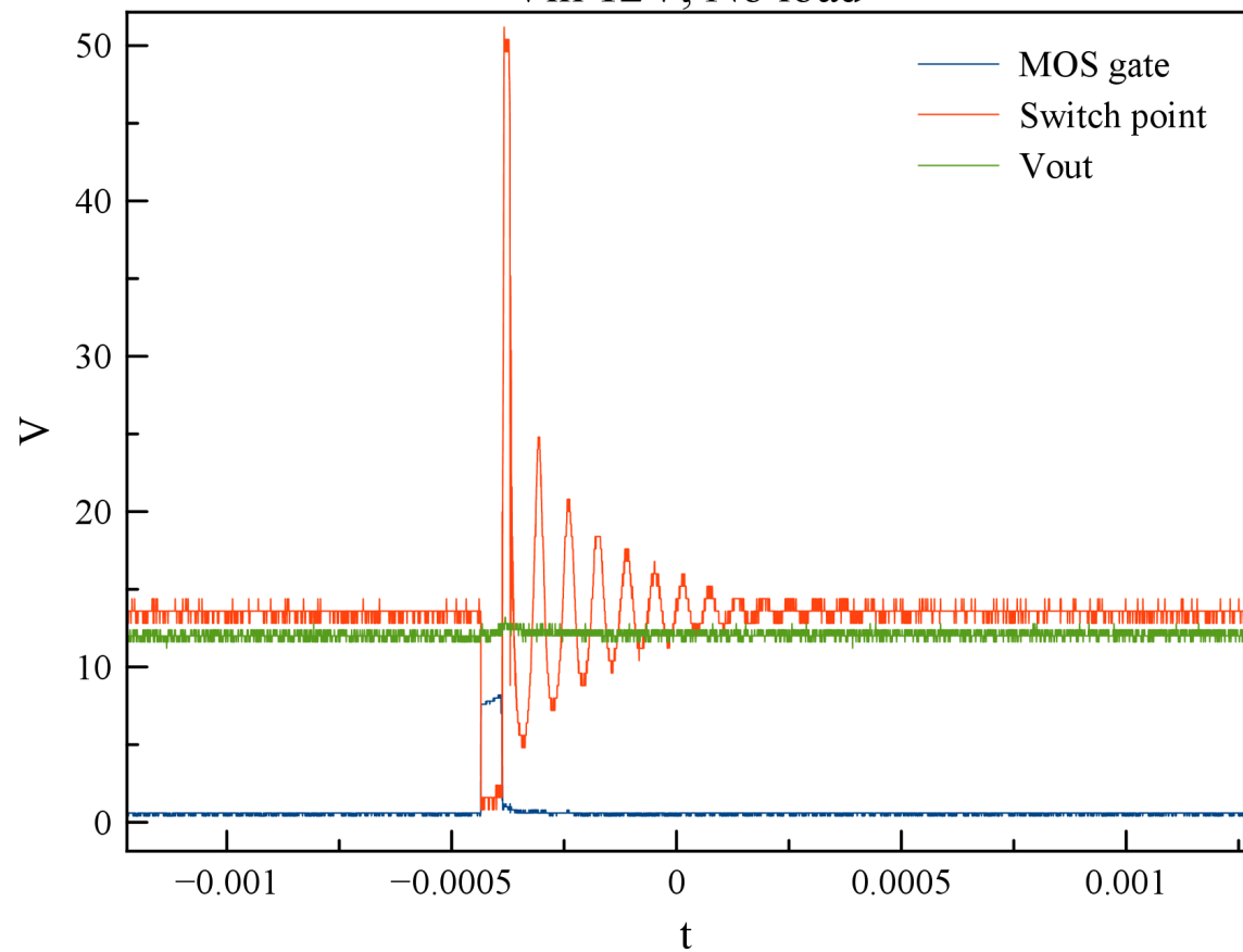
Vin 12V, No load
