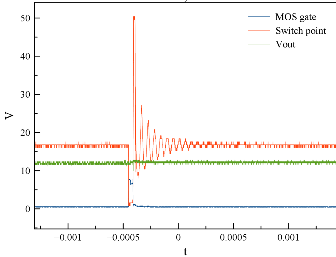
Vin 15V, No load
