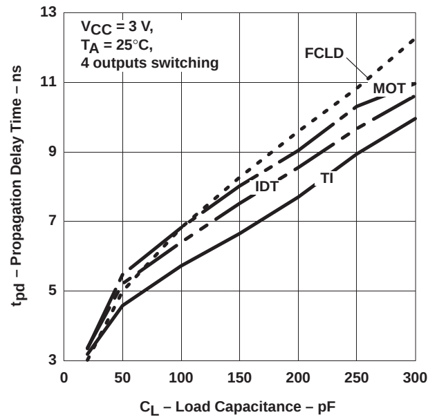
(d) '245 - t_{PHL}
