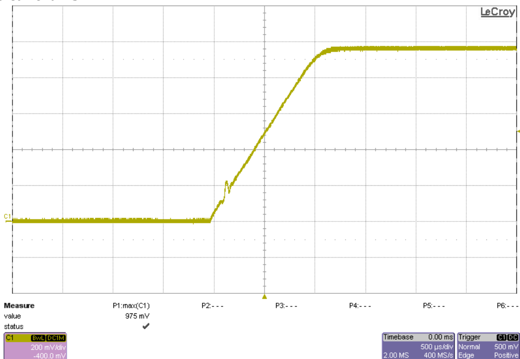
C1: VOUT_4A
