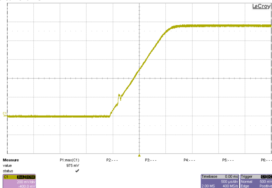
C1: VOUT_3A
