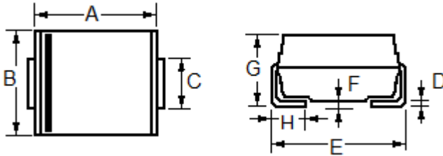
SMB (DO-214AA)
