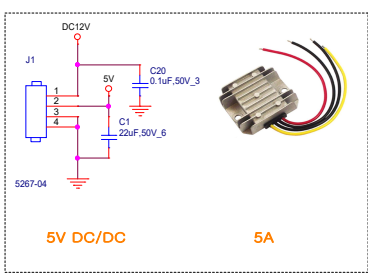
RASP PWR
