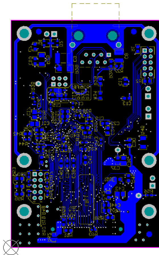
Figure 33. Altium Bottom Layer
