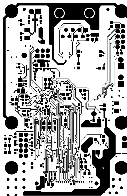
Figure 29. Bottom Layer
