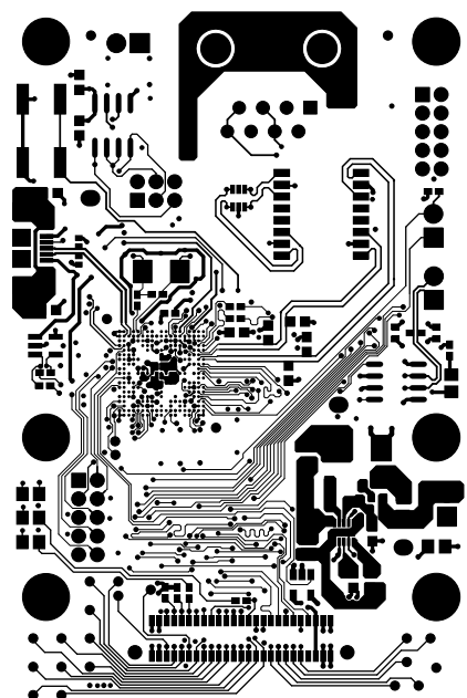
Figure 26. Top Layer
