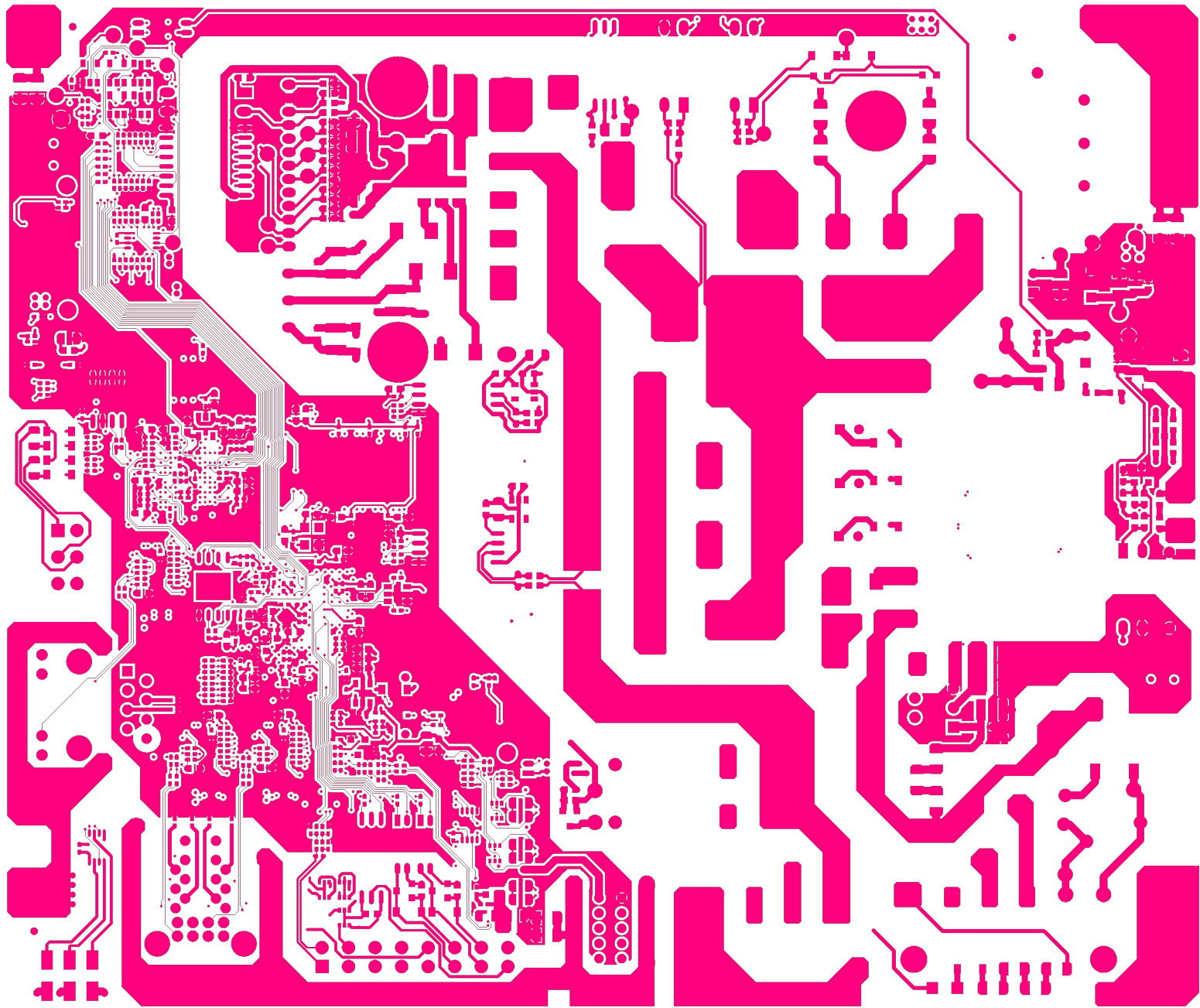
#6 BOTTOM LAYER
