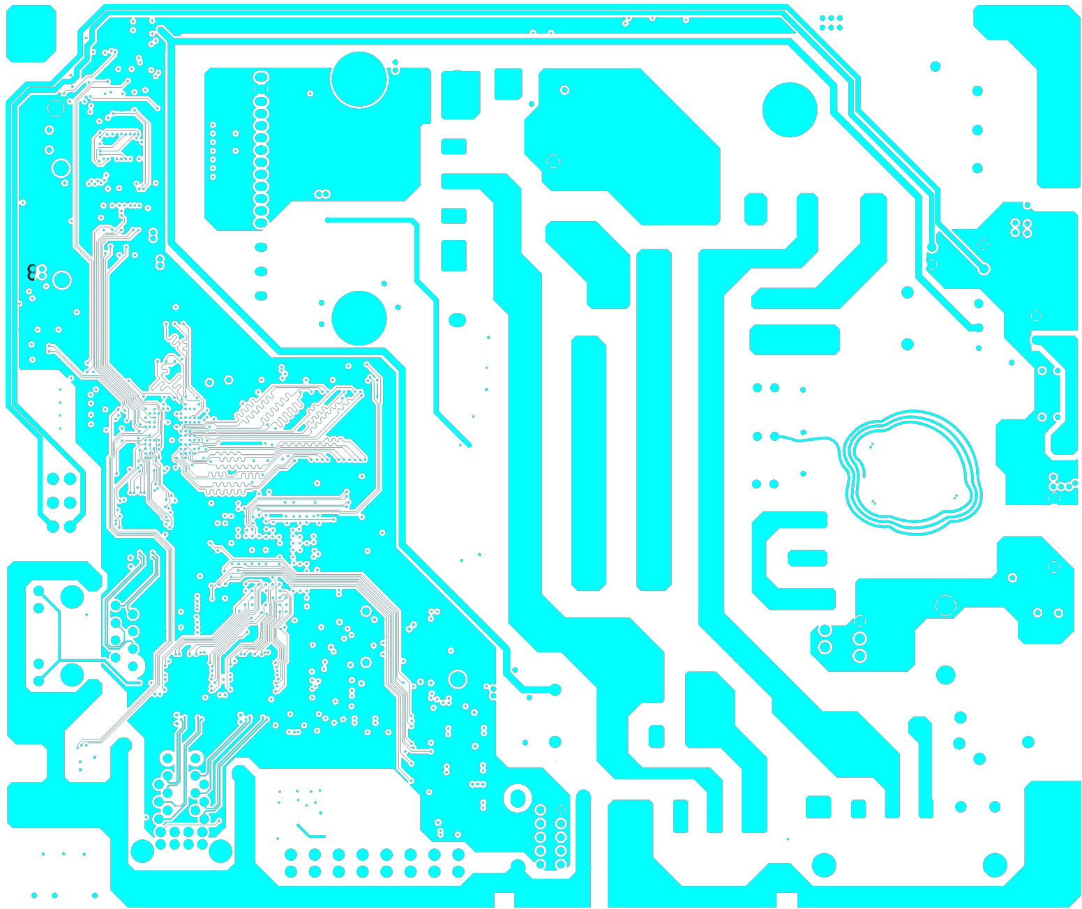
#3 INNER LAYER 3
