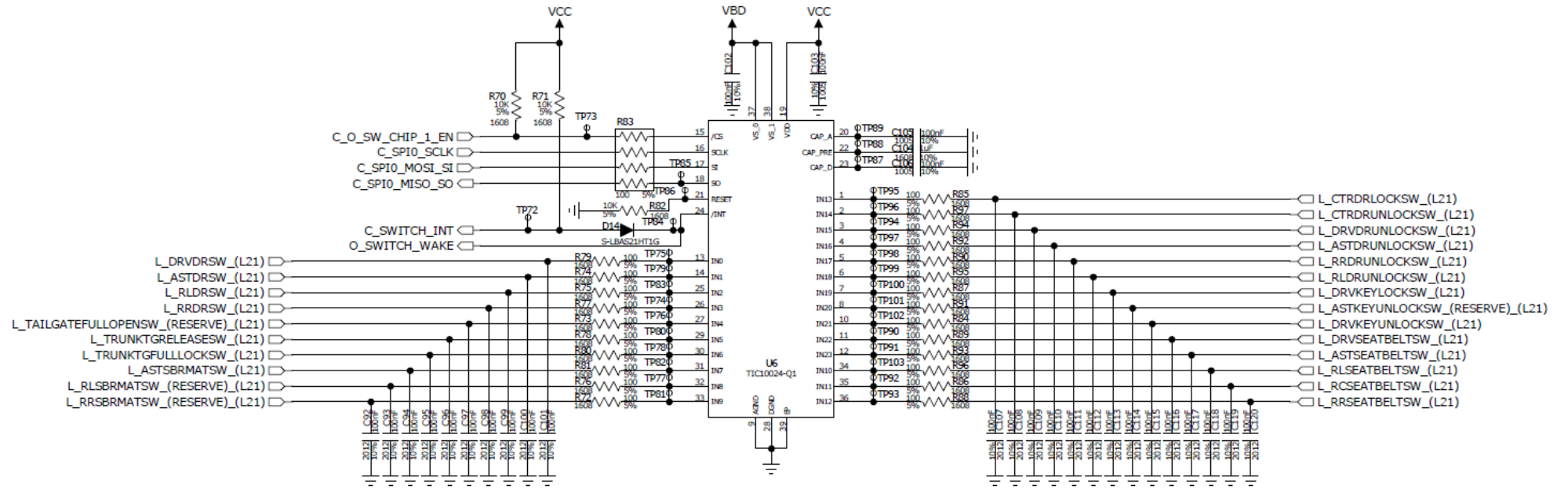
Schematic_TIC10024-Q1
