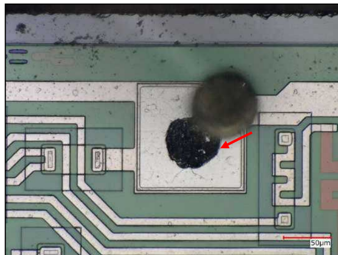
不具合品：図4.1㉒拡大 [ワイヤ剥がれが観察された]
