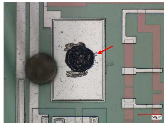
不具合品：図4.1㉓拡大 [ワイヤ剥がれが観察された]
