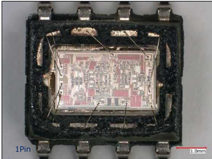
不具合品：開封部全体像
