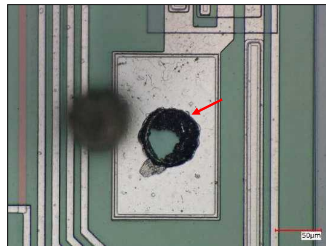
不具合品：図4.1⑥拡大 [ワイヤ剥がれが観察された]
