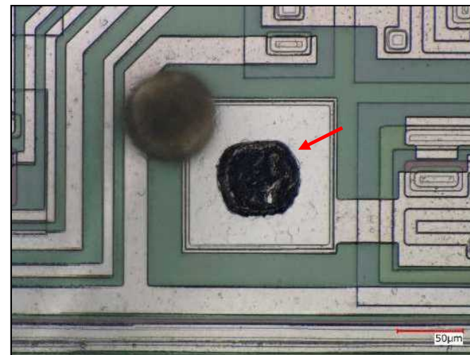
不具合品：図4.1③拡大 [ワイヤ剥がれが観察された]
