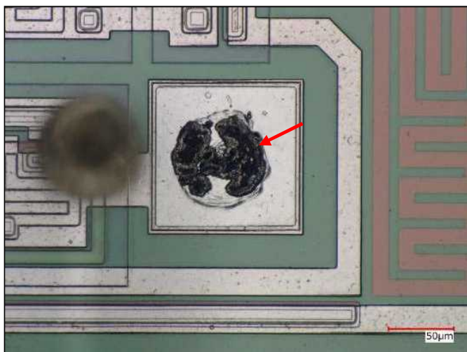
不具合品：図4.1④拡大 [ワイヤ剥がれが観察された]
