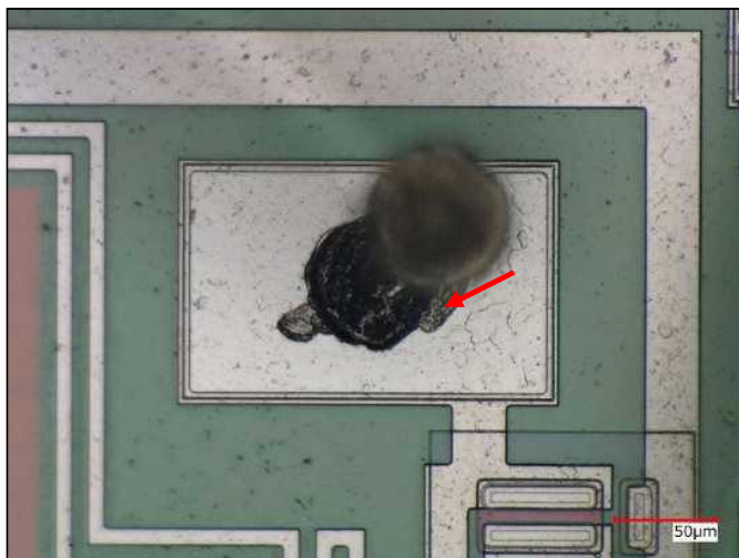
不具合品：図4.1㉑拡大 [ワイヤ剥がれが観察された]
