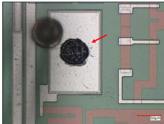
不具合品：図4.1②拡大 [ワイヤ剥がれが観察された]
