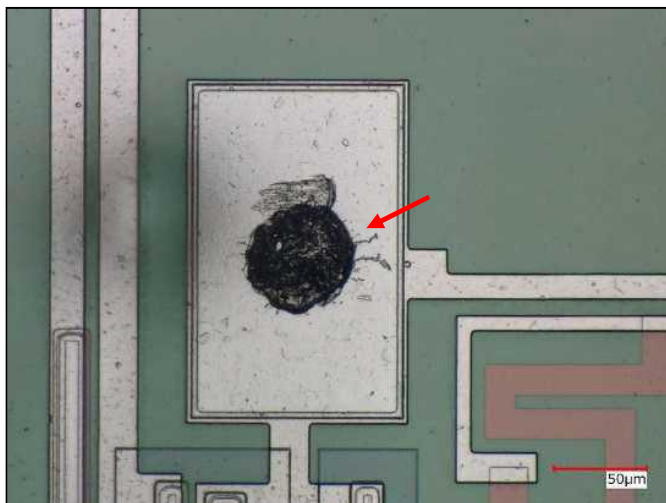
不具合品：図4.1①拡大 [ワイヤ剥がれが観察された]
