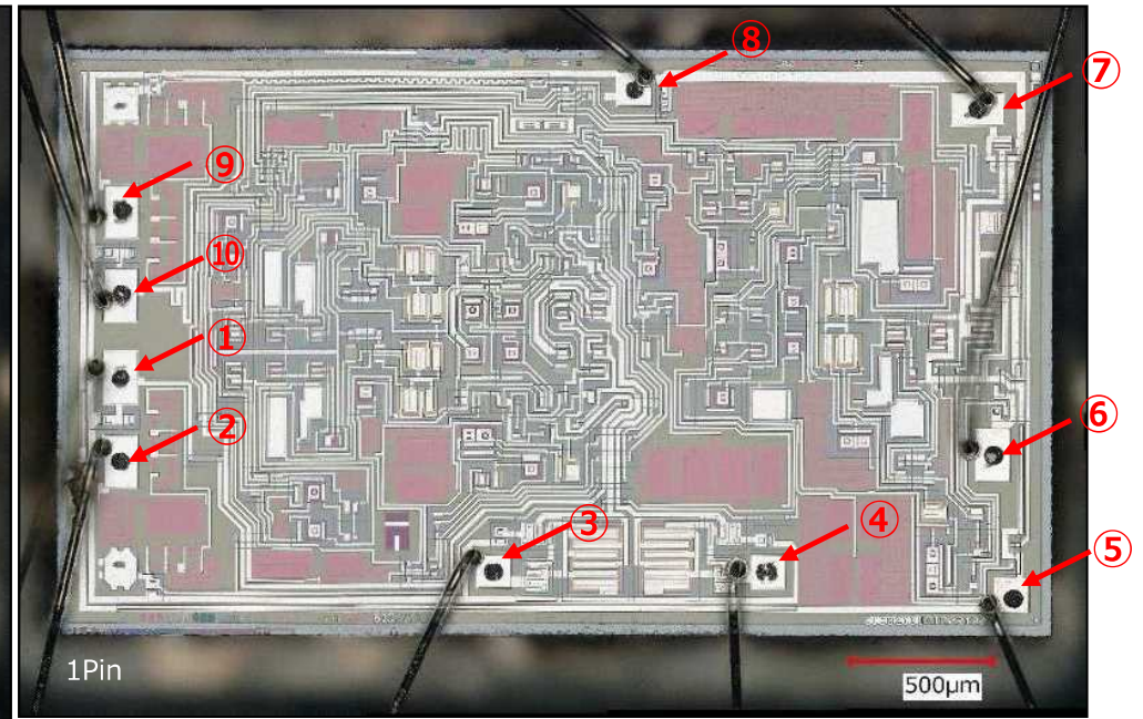
不具合品：チップ全体像（ワイヤ剥がれ状態確認後） [ワイヤ剥がれが観察された]
