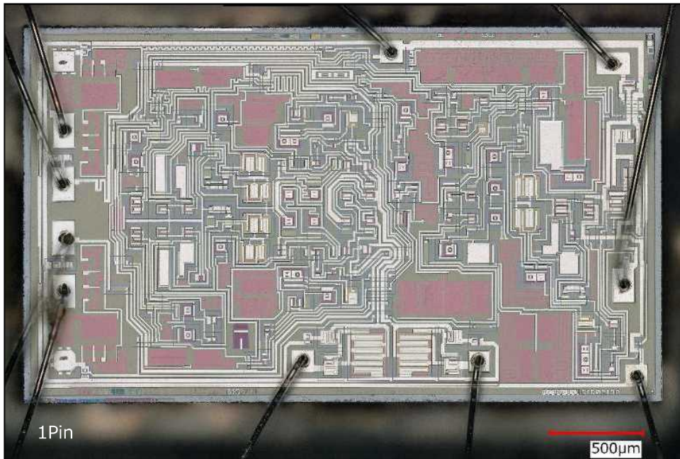
不具合品：チップ全体像（開封後）
