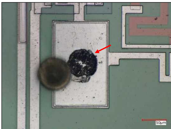
不具合品：図4.1㉔拡大 [ワイヤ剥がれが観察された]
