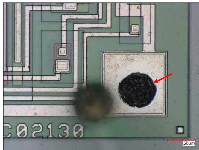
不具合品：図4.1⑤拡大 [ワイヤ剥がれが観察された]
