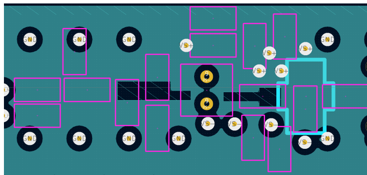
layer4 (VS+)
