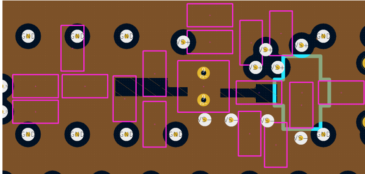
layer3 (VS-)
