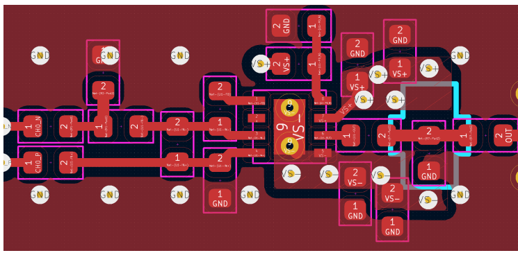
layer 1 (top)
