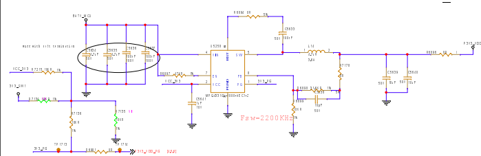
MCU&ADC POWER
