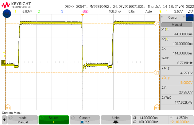
167 DP3M DUT2 AVCC 16V no Diode
