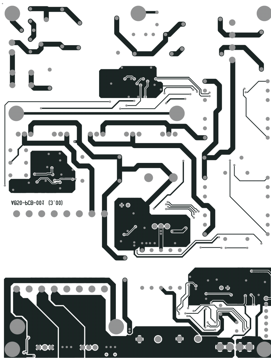
Figure 20. Bottom Layer
