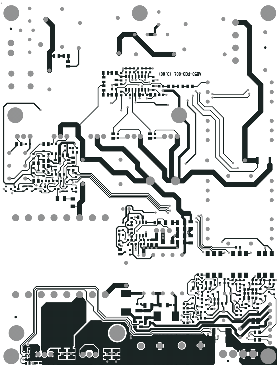
Figure 19. Top Layer
