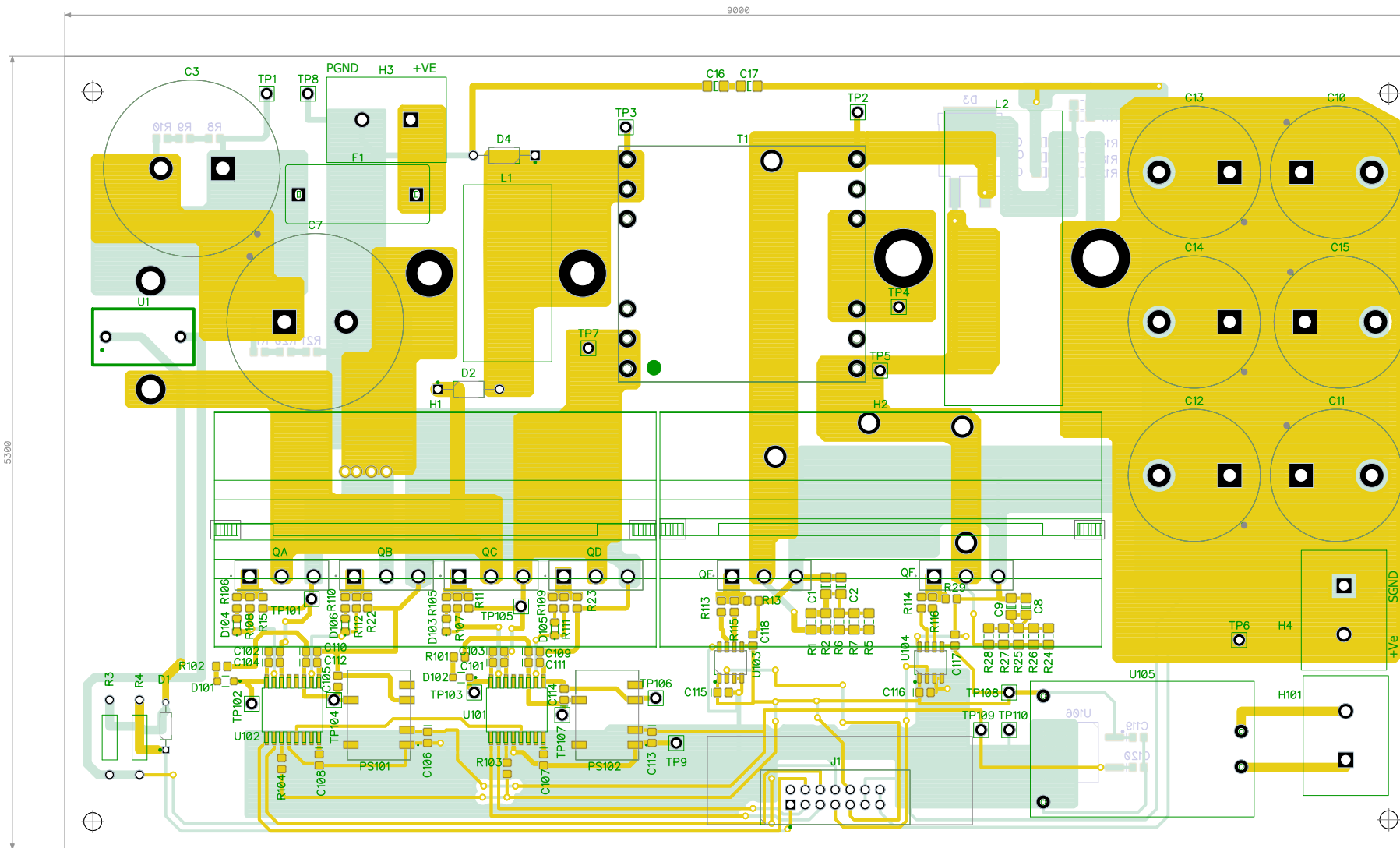
TOP LAYER
