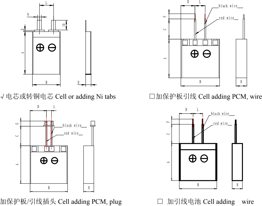
电芯外形尺寸参数表 Parameter:
