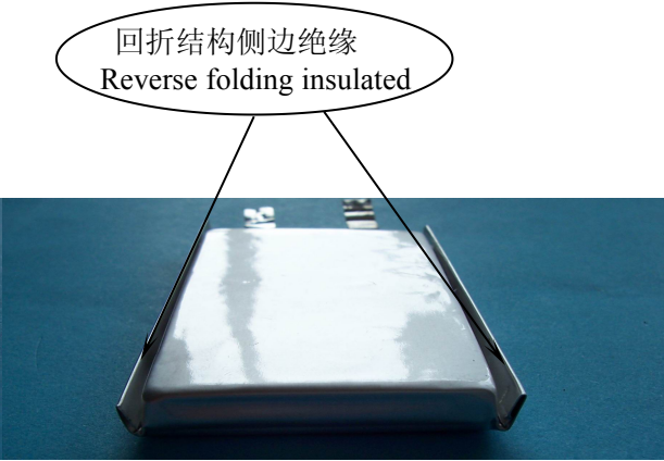
图 3：锂聚合物电芯双层折边示意图
