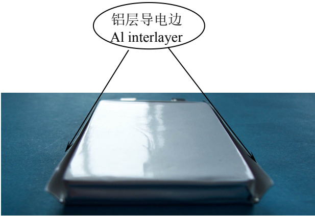
图 2：锂聚合物电芯单层折边示意图
