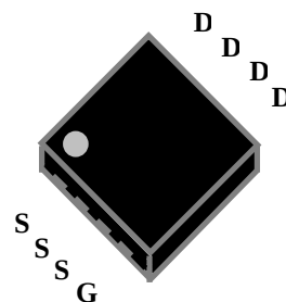
PMPAK ® 3 x 3
