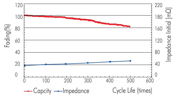
Cycle Life (23±2°C)
