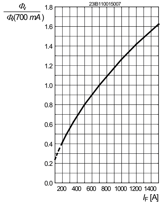
Relativer Lichtstrom 1) 2) 5) Seite 23 Relative Luminous Flux 1) 2) 5) page 23 \Phi_V/\Phi_V(700\text{ mA}) ; T_J = 25\text{ °C} ; ultra white
