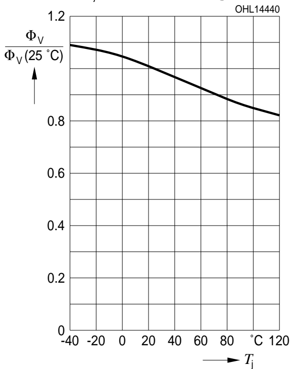
Relative Lichtstrom 1) 2) Seite 23 Relative Luminous Flux 1) 2) page 23 \Phi_V/\Phi_V(25\text{ °C}) = f(T_j); I_F = 700\text{ mA}; \text{true green}
