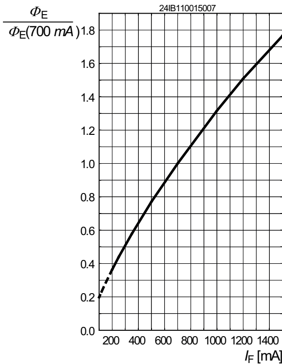
Relativer Strahlleistung 1) 2) 5) Seite 23 Relative Radiant Power 1) 2) 5) page 23 \Phi_E/\Phi_E(700\text{ mA}) ; T_J = 25\text{ °C} ; deep blue
