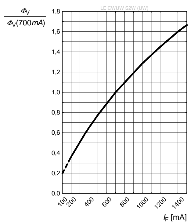
Relativer Lichtstrom 1) 2) 5) Seite 23 Relative Luminous Flux 1) 2) 5) page 23 \Phi_V/\Phi_V(700\text{ mA}) ; T_J = 25\text{ °C} ; ultra white
