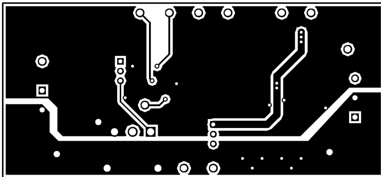
Figure 21. Bottom Layer
