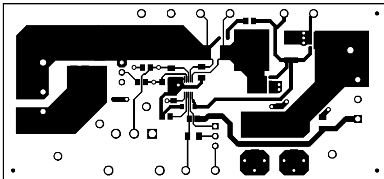
Figure 20. Top Layer
