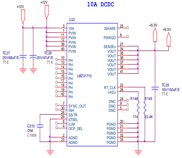
12V 입력 DC-DC 회로
