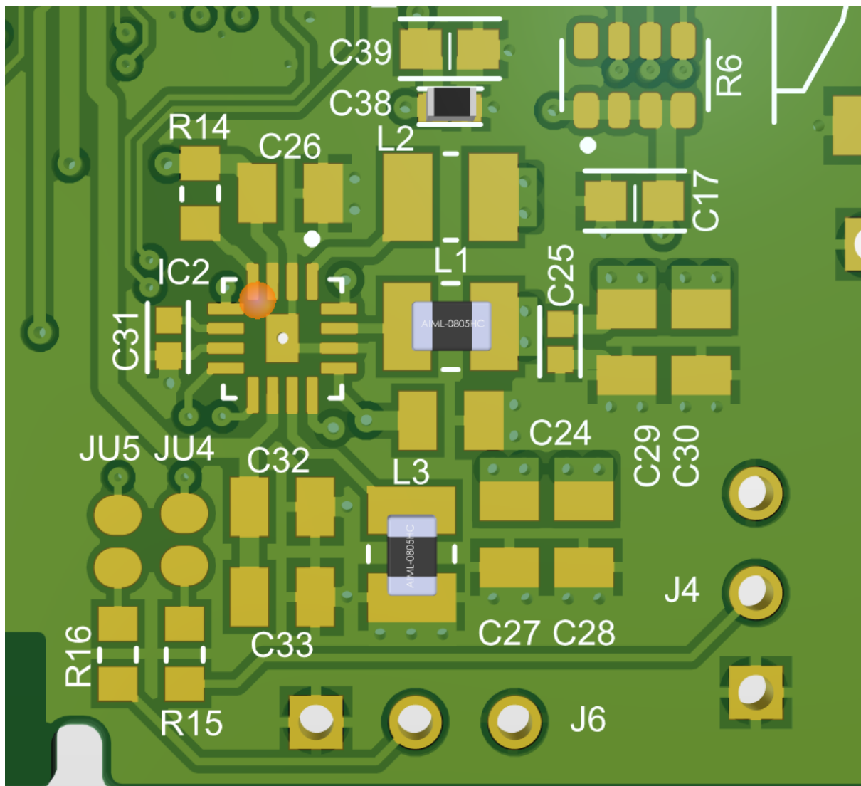
3D Top Layer
