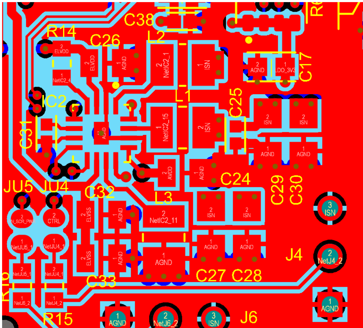
Bottom Layer
