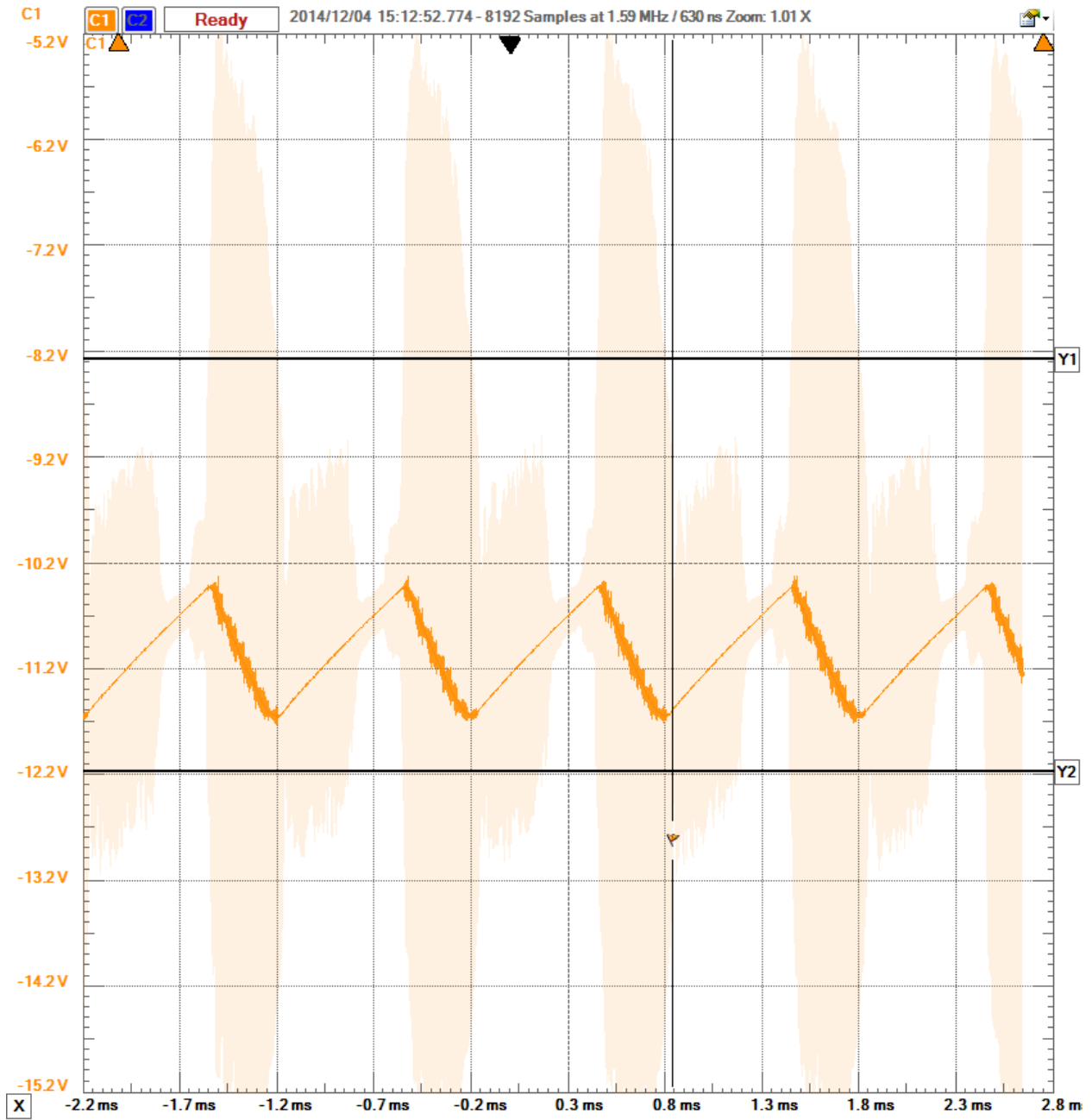
V_{out} node 1kHz 1 V_{pp} slow ripple.
