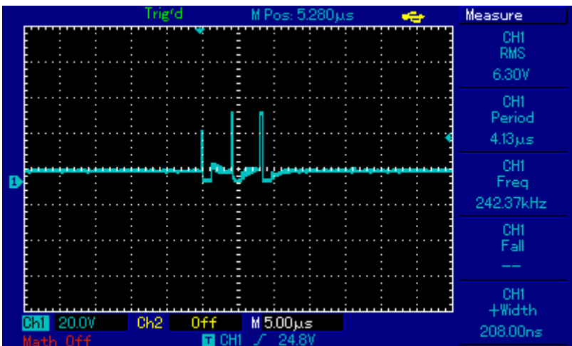
SW_without_load_40v_2
