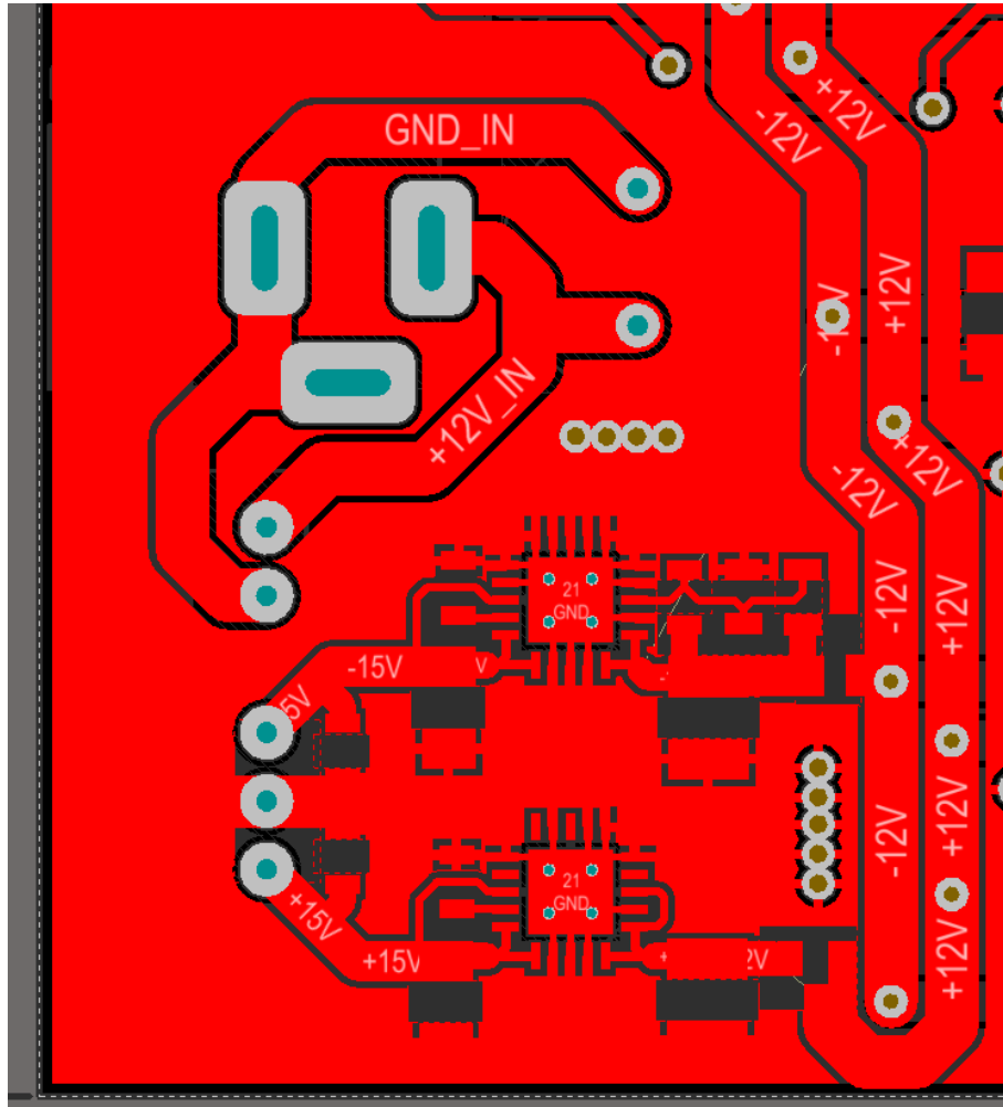
TOP LAYER
