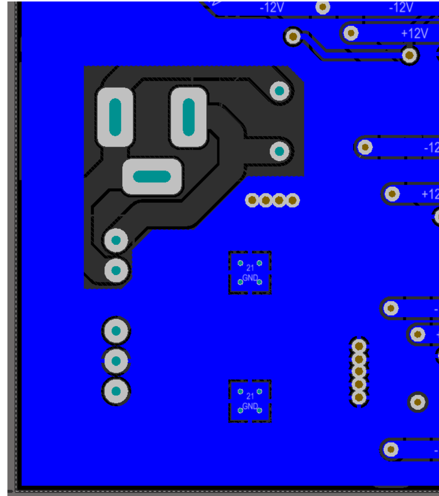
BOTTOM LAYER
