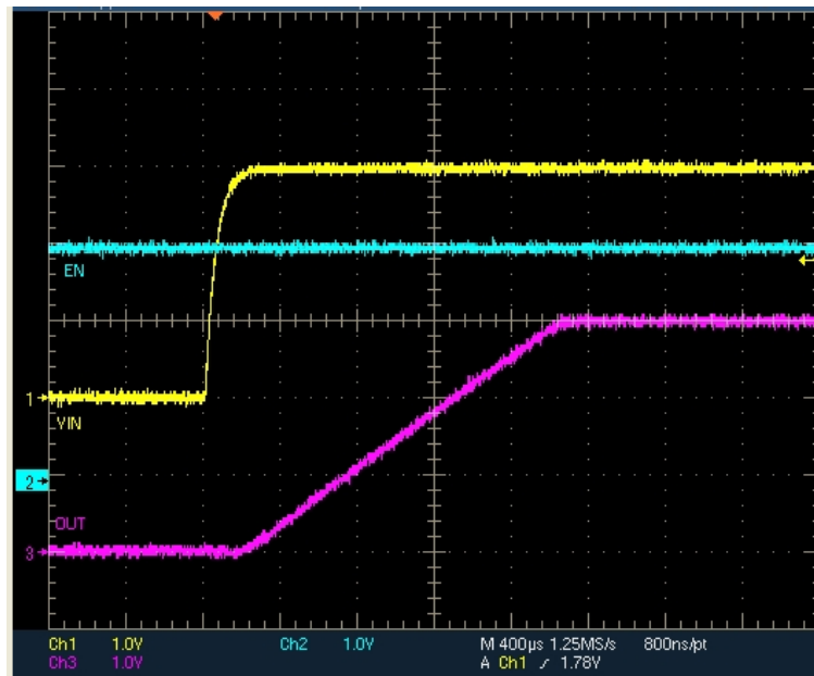
(Sequence-2) EN -> VIN
