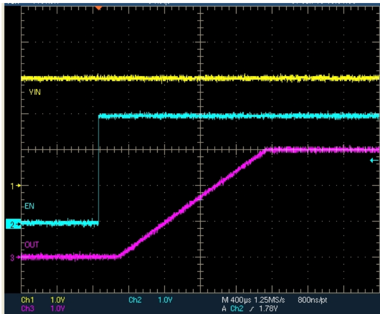
(Sequence-1) VIN -> EN
