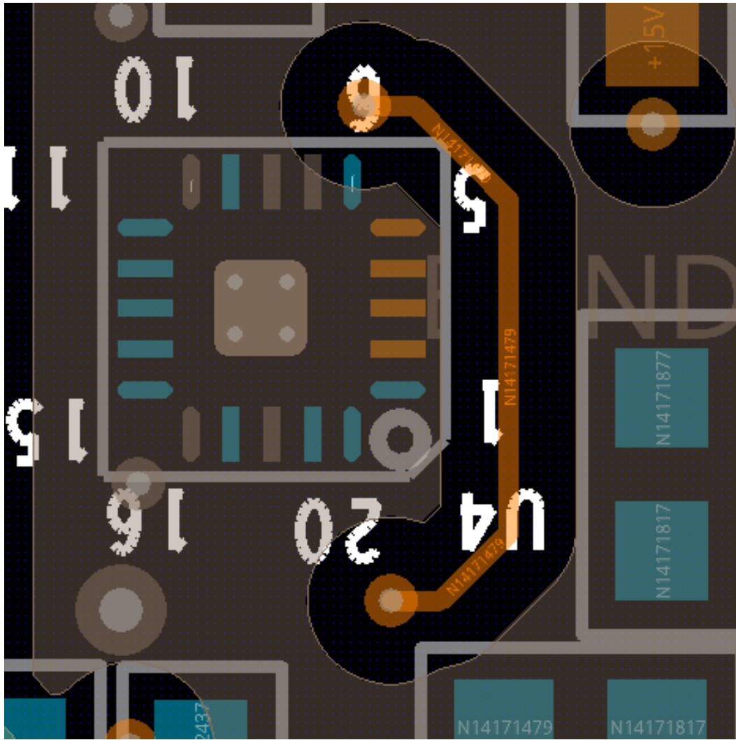
Inner Layer 2
