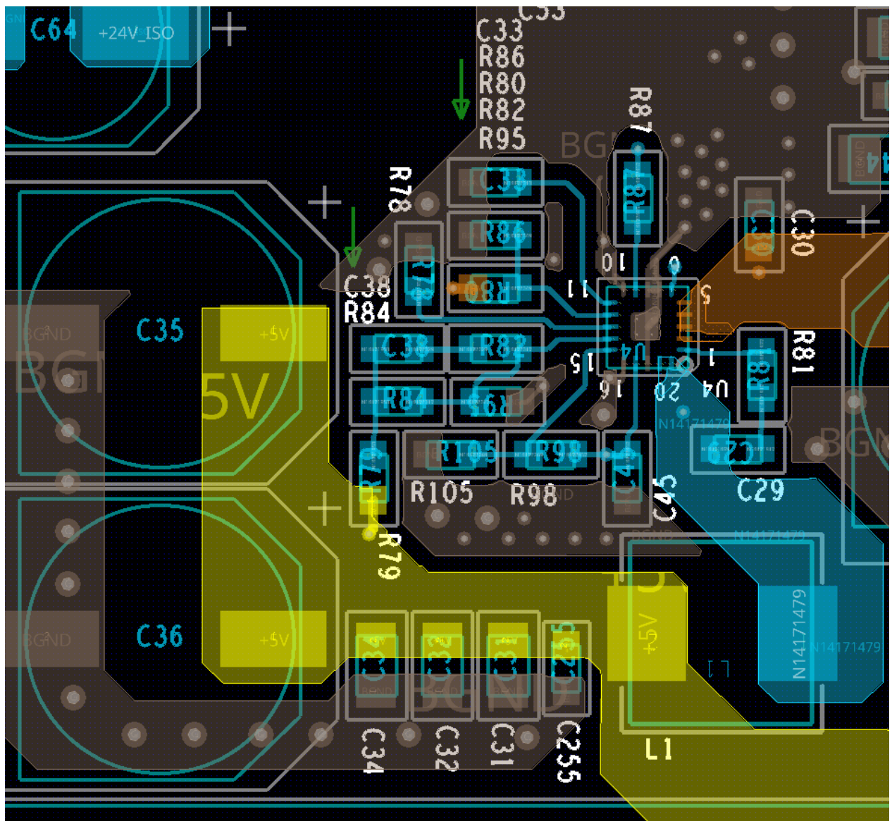
TOP Layer
