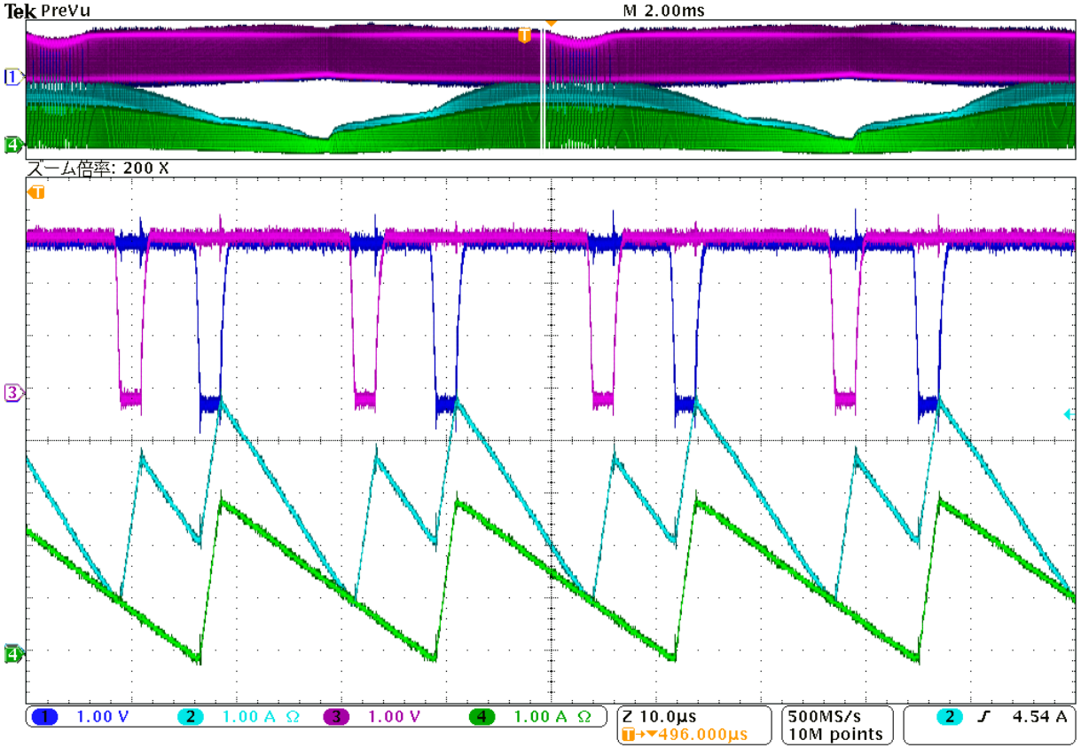
UCC28063A Waveform②-2
