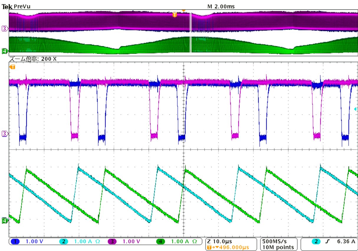
UCC28063A Waveform②-1
