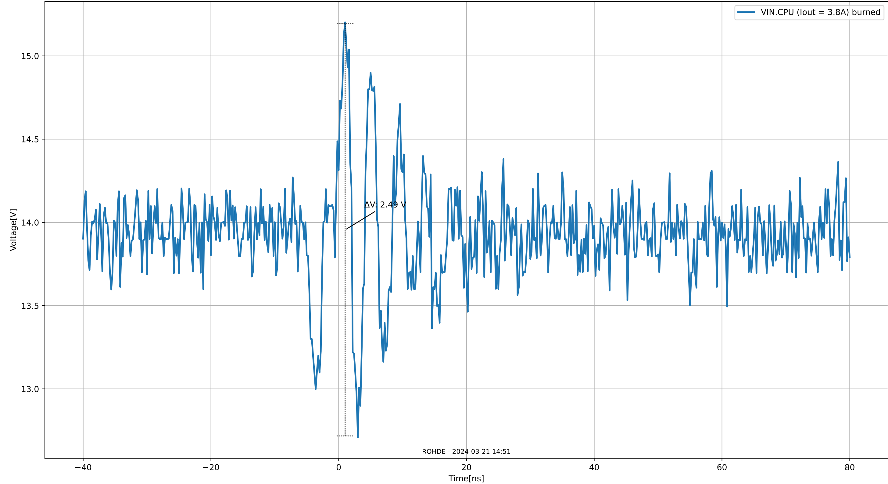
Vin [XF-PSU REV A] @ 500MHz
