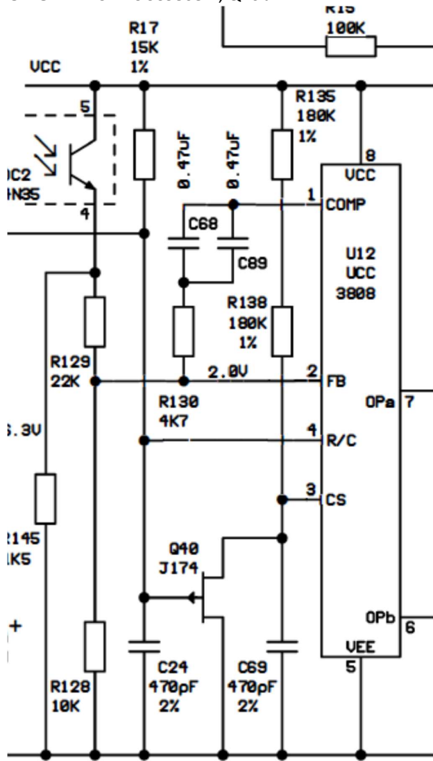
ORIGINAL: U12 UCC3808-1, Q40 J177
