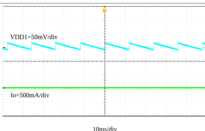
Figure 41. VDD1 Output Voltage Ripple, I_{OUT} = 0 A
