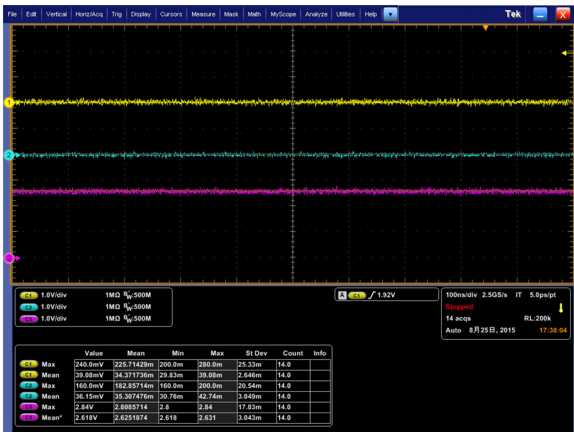
Fig. 3. CS1 (CH1) , CS2 (CH2) , Slope 端子 (CH3) 電圧波形 (横軸 100nsec./div.)
