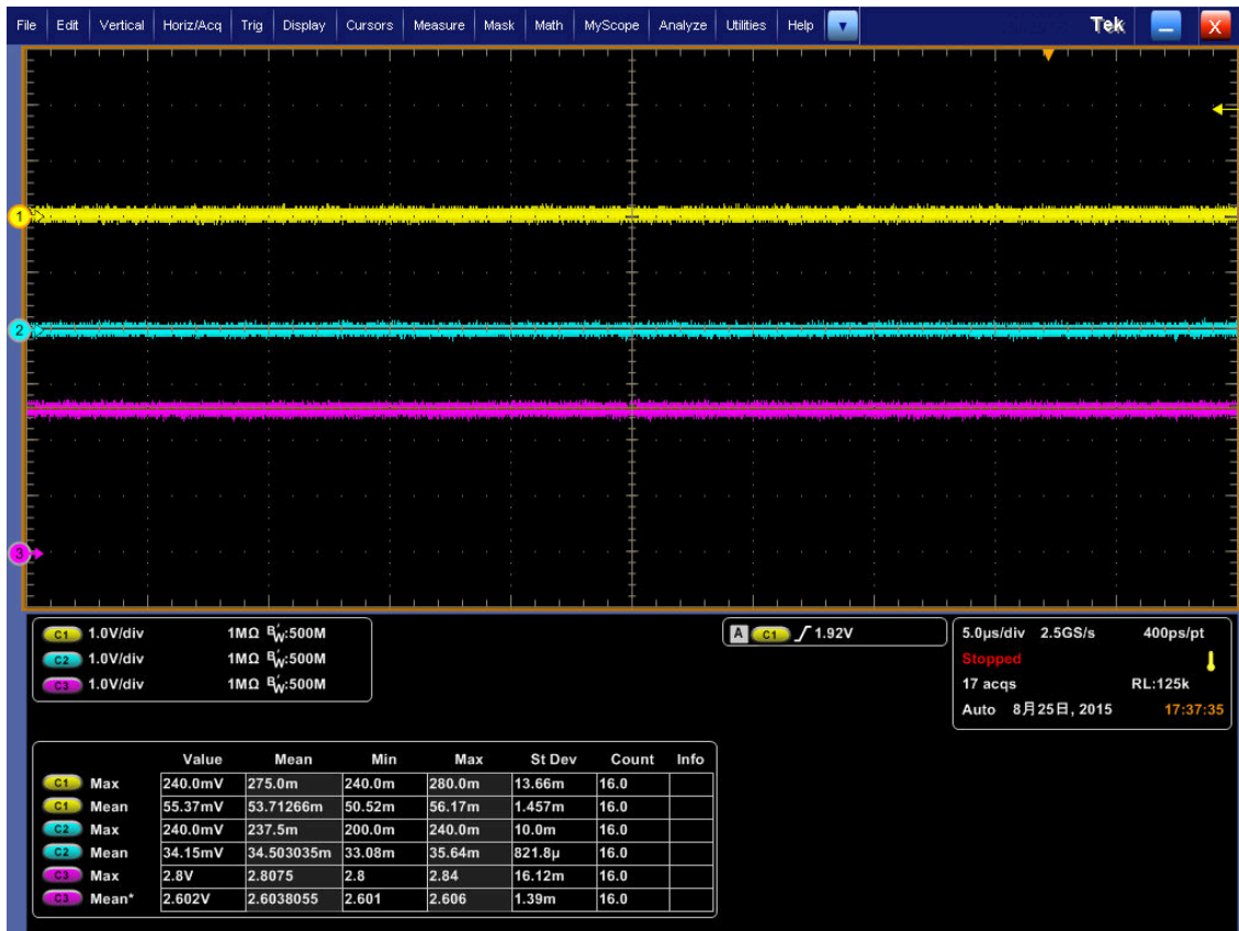
Fig. 2. CS1 (CH1) , CS2 (CH2) , Slope 端子 (CH3) 電圧波形 (横軸 5µsec./div.)
