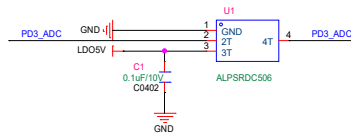
电位计
