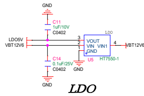
LDO
