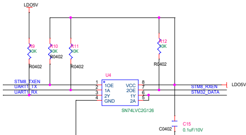
逻辑转换
