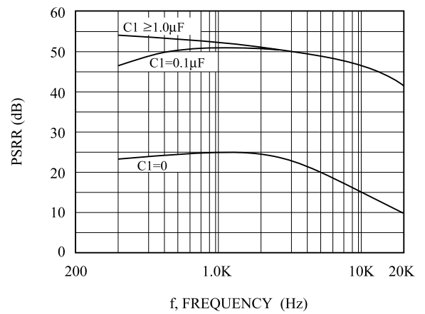
FIGURE5-C2=5.0μF
