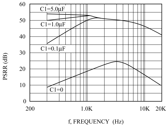
FIGURE6-C2=1.0μF
