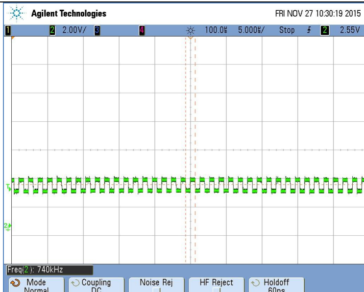
Audio play 명령 실행 후 상태 (BCLK)
