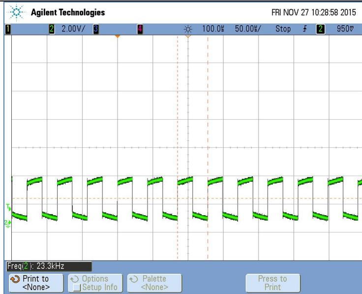
Audio play 명령 실행 전 상태 (BCLK)
