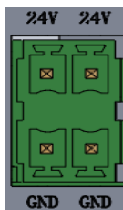
图 5.2 直流供电接线图
