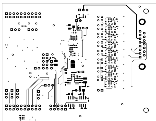
Figure 41. Bottom Layer
