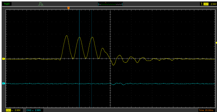
GPMCCLKDIVIDER:3
