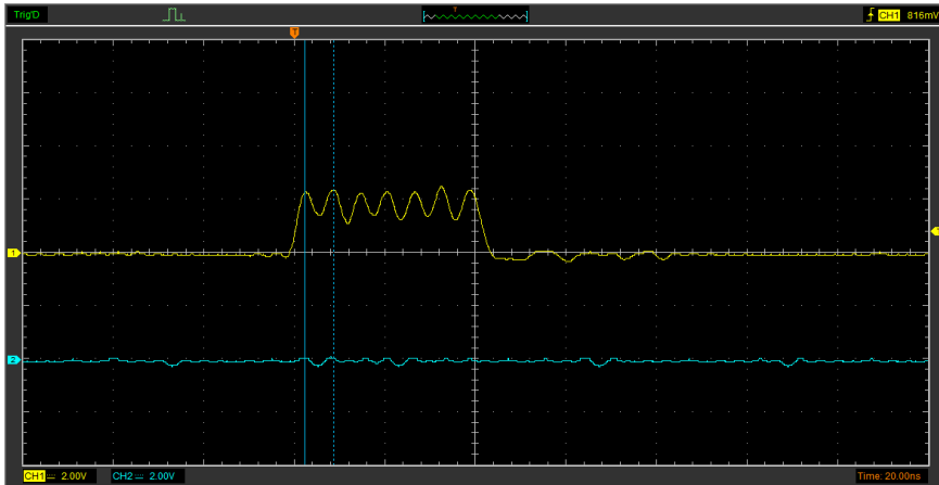
GPMCCLKDIVIDER:2
