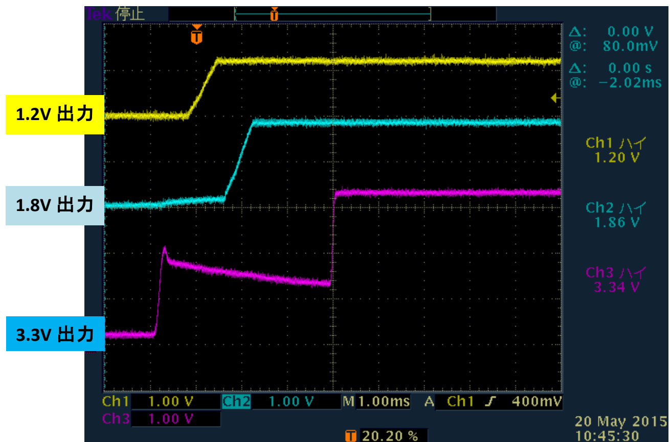
波形② 電圧は正常だが、3.3V が先に立ち上がる場合
