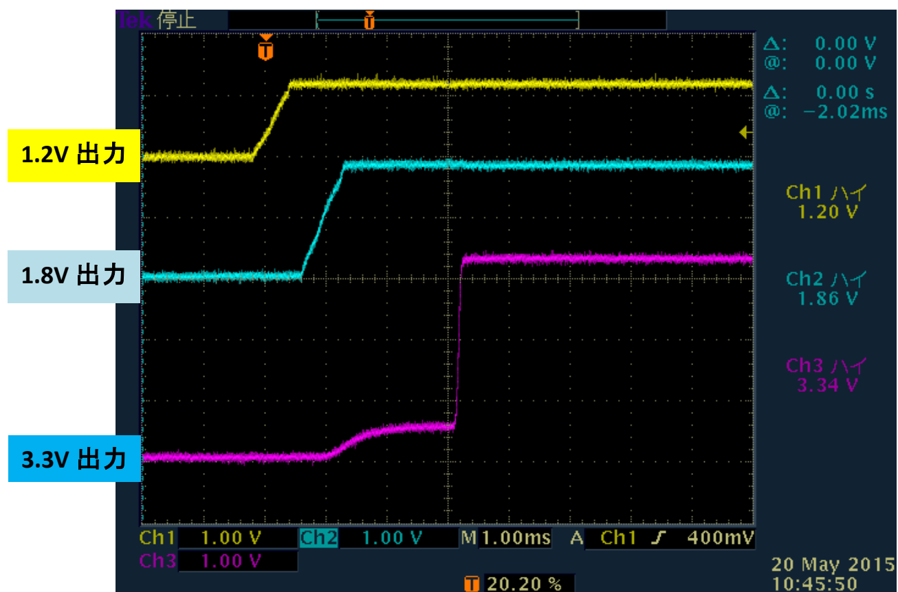
波形① 正常時
