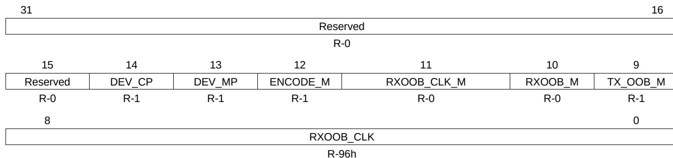
Figure 29-15. Global Parameter 2 Register (GPARAM2R)
