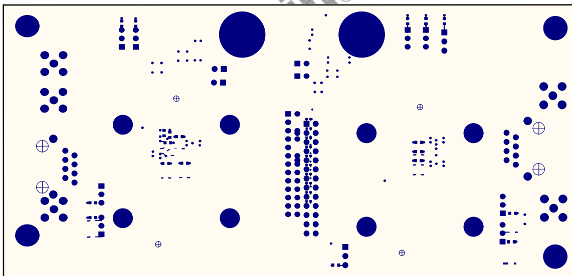
Bottom Layer
