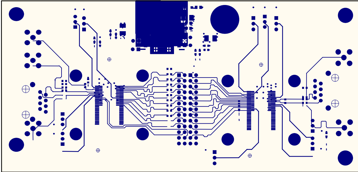
Top
