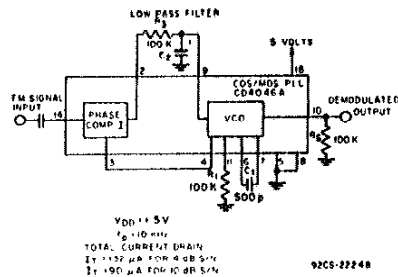
Fig. 10— FM demodulator.
